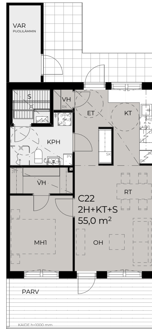
POHJAPIIRUSTUS
