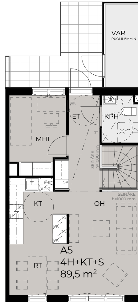
2. KRS POHJAPIIRUSTUS
