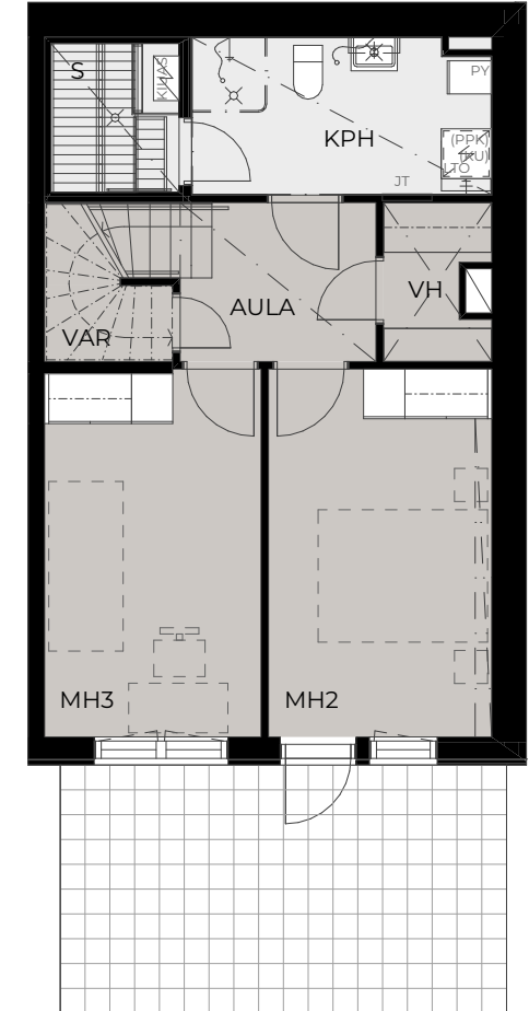
1. KRS POHJAPIIRUSTUS
