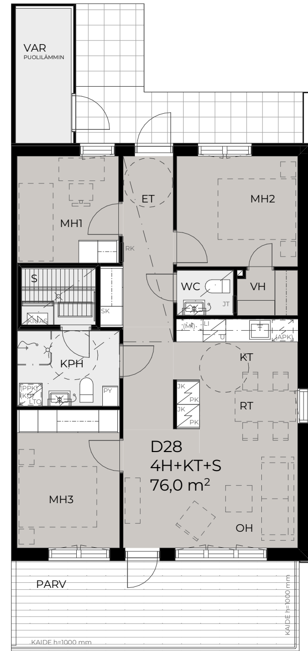
POHJAPIIRUSTUS
