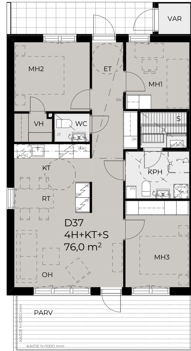
POHJAPIIRUSTUS
