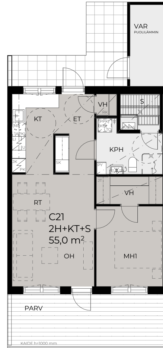
POHJAPIIRUSTUS
