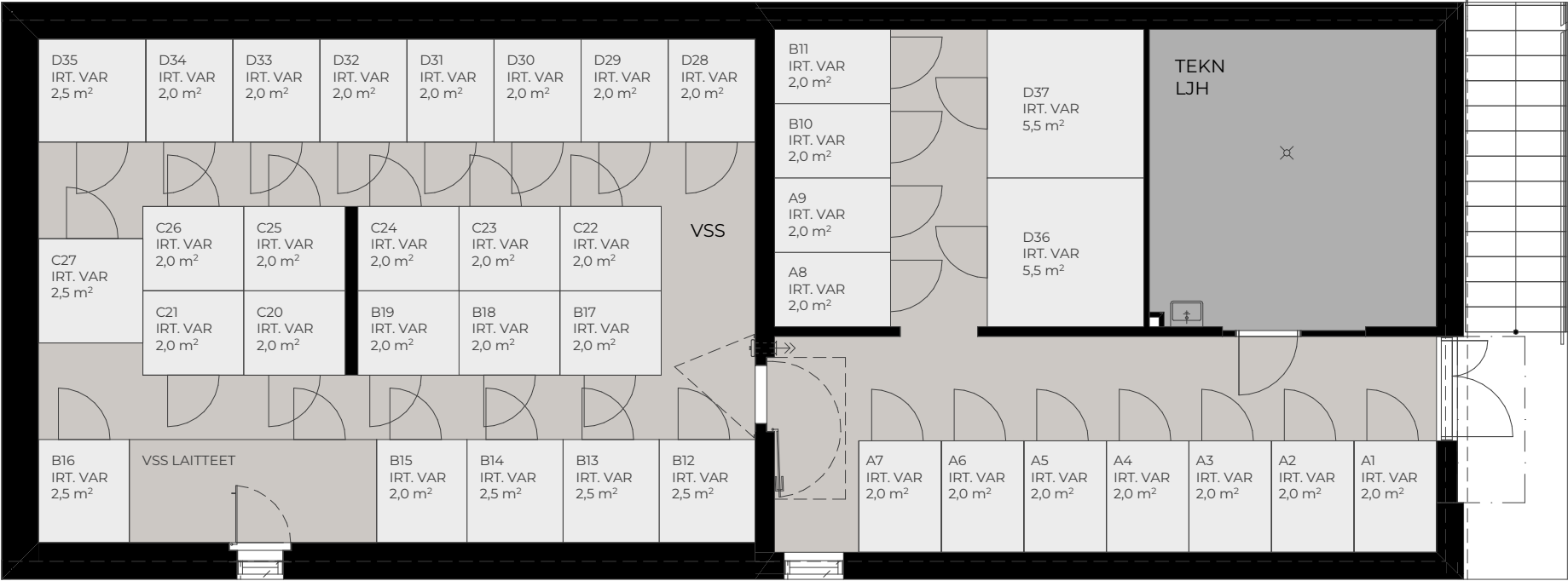
KELLARIKERROS POHJAPIIRUSTUS TALO C
