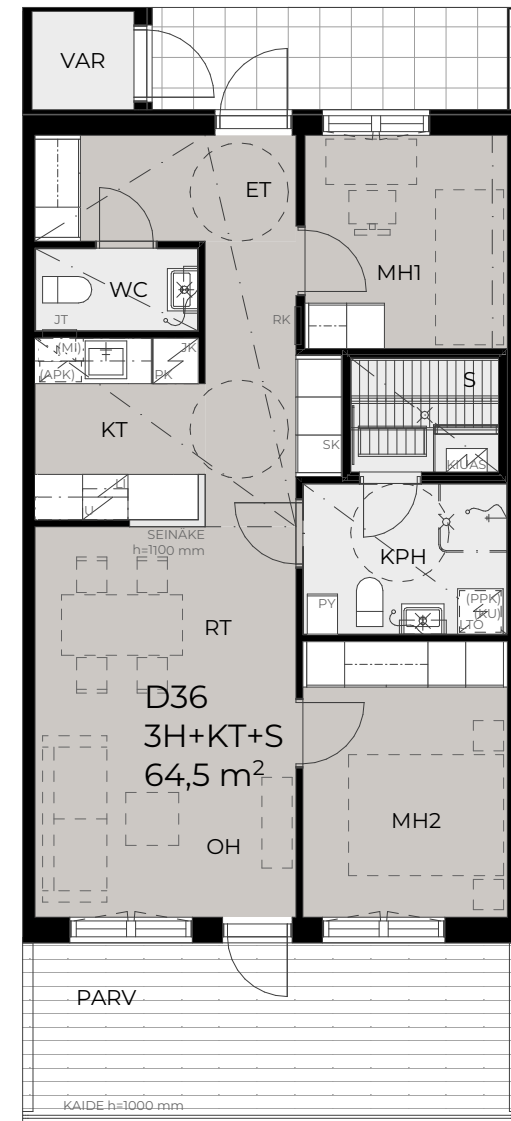
POHJAPIIRUSTUS
