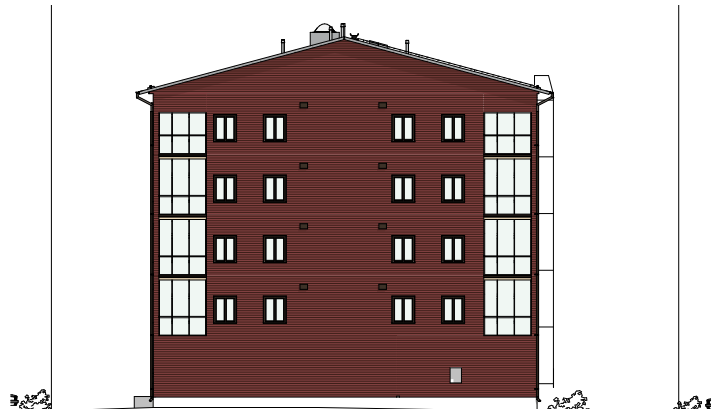
Julkisivu luoteeseen, 1:400
